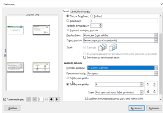
Εικόνα 4.24. Επιλογές Εκτύπωσης
